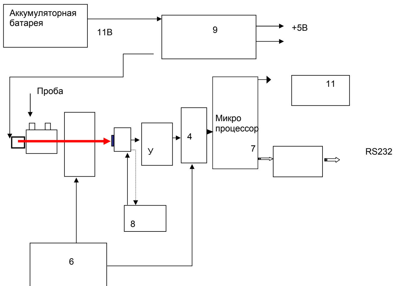
Рисунок 1 - Функциональная схема ГА
